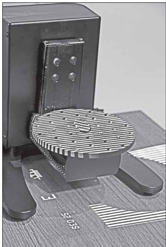
Монета на рабочем столике ювелирного сканера
